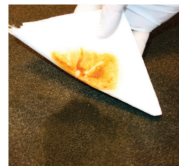
BLOT
